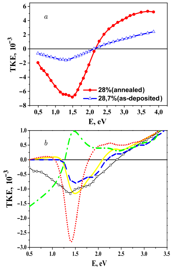
Рис. 6. (В цвете онлайн) a ) Спектральные зависимости ТКЕ нанокompозита (CoFeZr)_x(Al_2O_3)_{100-x} при x = 28 ат. % в исходном состоянии и после отжига (эксперимент). b ) Результаты расчета ТКЕ для нанокompозита (CoFeZr)_x(Al_2O_3)_{100-x} при x = 18.5 ат. % в рамках СМГ без учета размерного эффекта (зеленый штрихпунктир) и при учете размерного эффекта для гранул размером r_0 = 1.0 нм (синие штрихи), r_0 = 1.2 нм (сплошная желтая линия) и r_0 = 2.0 нм (красные точки). Данные взяты из работы [14]
