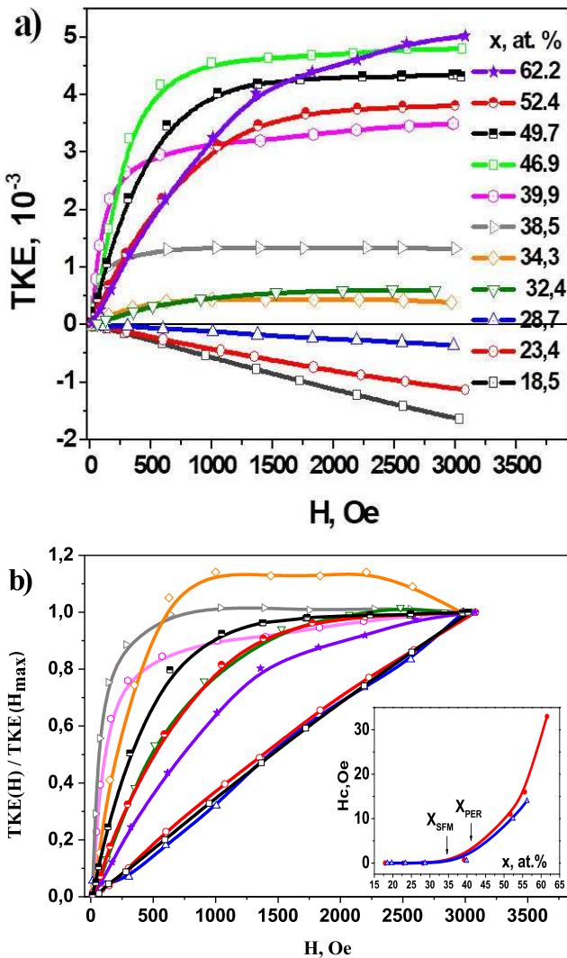
Рис. 3. (В цвете онлайн) Полевые зависимости ТКЕ для нанокompозита (\text{CoFeZr})_x(\text{Al}_2\text{O}_3)_{100-x} в исходном состоянии при E = 1.97 эВ (a) и нормированные на сигнал в максимальном поле, \text{TKE}(H)/\text{TKE}(H_{\text{max}}) (b). На вставке к рис. 3b показана концентрационная зависимость коэрцитивной силы H_c , полученная из магнитных измерений; величина x_{\text{per}} определена из транспортных измерений, а x_{\text{SFM}} соответствует концентрации, при которой СФМ-состояния были найдены из МО-измерений. Данные взяты из работы [19]
