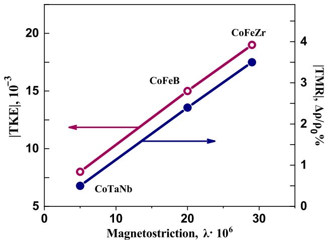
Рис. 5. Корреляция между ТКЕ нанокompозитов, магнитоупругостью ферромагнитной компоненты и туннельным магнитосопротивлением (ТМР). Данные взяты из работы [23]
