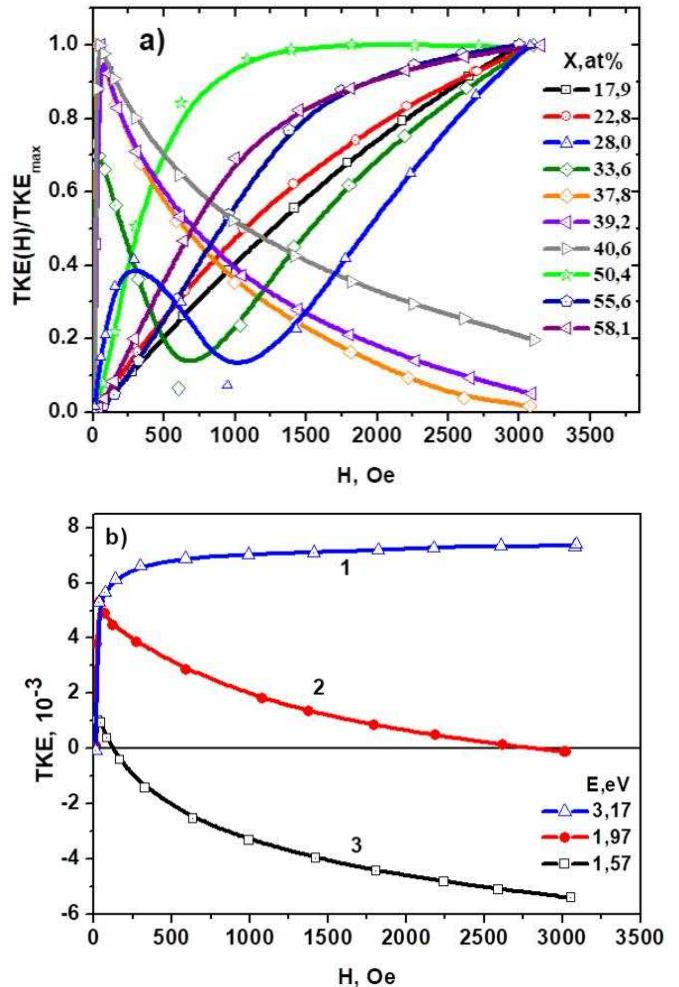
Рис. 4. (В цвете онлайн) Нормированные полевые зависимости \text{TKE}/\text{TKE}_{\text{max}} для отожженных нанокompозитов (\text{CoFeZr})_x(\text{Al}_2\text{O}_3)_{100-x} при E = 1.97 эВ (a) и полевые зависимости ТКЕ при энергиях фотонов 1.57, 1.97 и 3.17 эВ (b). Данные взяты из работы [19]
