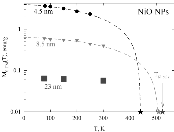
Рис. 3. (В цвете онлайн) Температурная эволюция величины M_{S\_FM} (символы), полученная из результатов обработки зависимостей M(H) (рис. 2) для серии образцов NiO. Линии построены по выражению (3) при a = 1.75 и a = 1.5 для образцов NiO 4.5 и 8.5 нм, соответственно; «звезды» на оси абсцисс соответствуют температурам, при которых значения выражения (3) для величин M_{S\_FM} образцов NiO 4.5 и 8.5 нм становятся равными нулю; также обозначена температура Нееля T_{N\_bulk} объемного NiO
