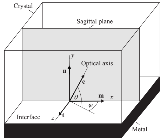
Рис. 1. Волновая геометрия распространения в координатной системе
