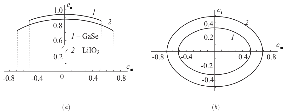
Рис. 6. Проекция границ запрещенных зон на плоскости (\mathbf{m}, \mathbf{n}) (а) и (\mathbf{m}, \mathbf{t}) (б) для отрицательных кристаллов GaSe (1) и LiIO 3 (2) при \lambda_{vac} = 1.0 мкм
