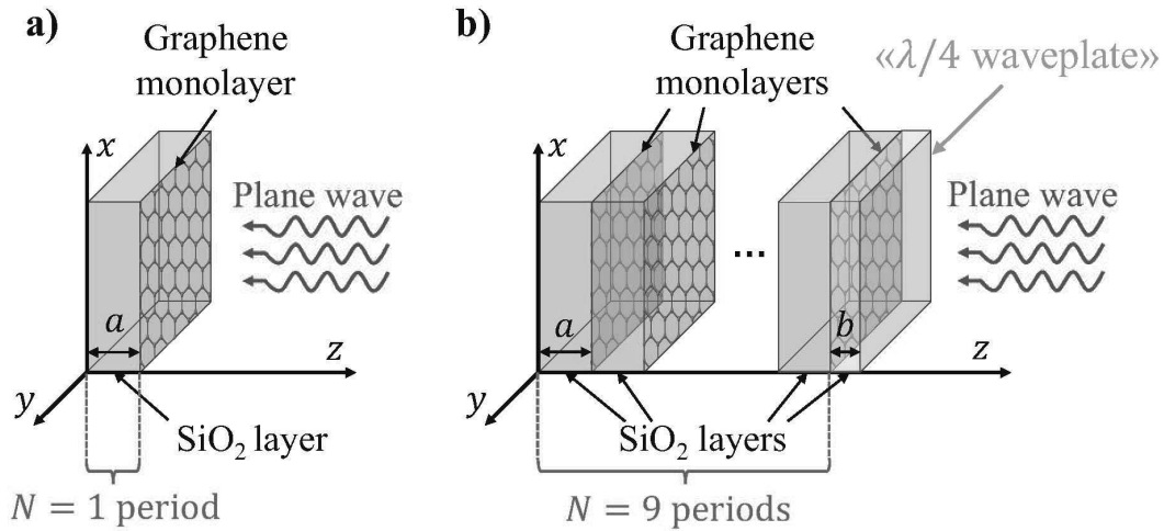
Рис. 1. Характерный вид исследуемой структуры диэлектрик–графен для детектирования квазимонохроматического излучения (a) и широкополосного излучения (b). Одним периодом структуры считается бислой графен + диэлектрическая подложка из SiO 2
