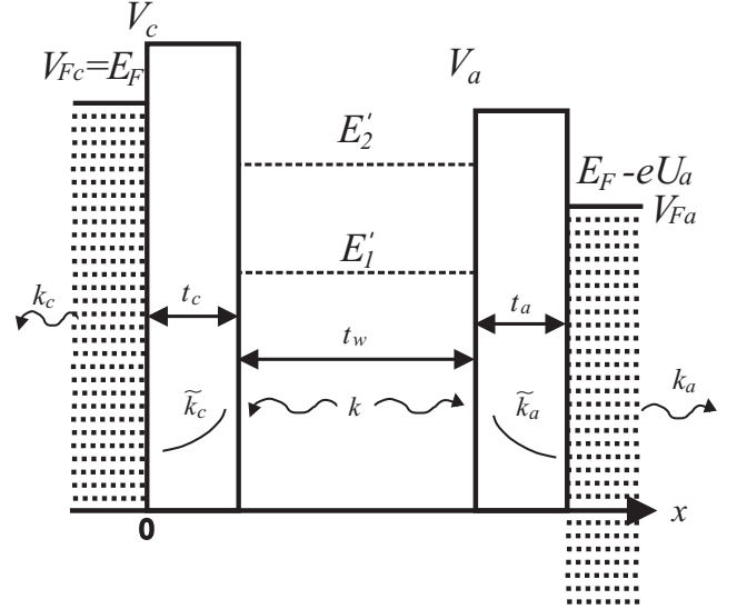
Рис. 2. Схематическое распределение потенциала V в одноячейной РТС при U_g = E_F/e . Штриховыми линиями обозначены уровни на катоде, аноде и два метастабильных уровня
