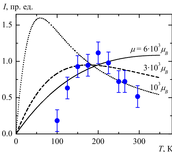
Рис. 7. Температурная зависимость интегральной интенсивности I(T) линии ЭПР ( g \approx 4 ) для пленки \text{Ni}_{50}(\text{Al}_2\text{O}_3)_{50} . Символы — экспериментальные данные на частоте f \approx 18 ГГц, линии — расчет в модели «гигантского спина» с разными значениями магнитного момента гранул \mu
