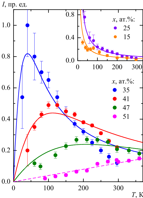
Рис. 6. Температурные зависимости интегральной интенсивности I(T) линии ЭПР ( g \approx 4 ) для пленок нанокompозитов (\text{CoFeB})_x(\text{Al}_2\text{O}_3)_{100-x} . Символы — экспериментальные данные на частоте f \approx 25 ГГц, сплошные линии — расчет в модели «гигантского спина», штрихи — линейная зависимость. Линии на вставке — закон Кюри I(T) \propto 1/T
