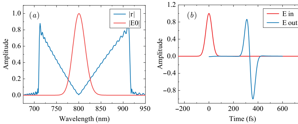
Рис. 2. a — Спектр модуля коэффициента отражения в сравнении со спектром падающего импульса, b — временные профили действительной части падающего и отраженного от данного ФК импульсов
