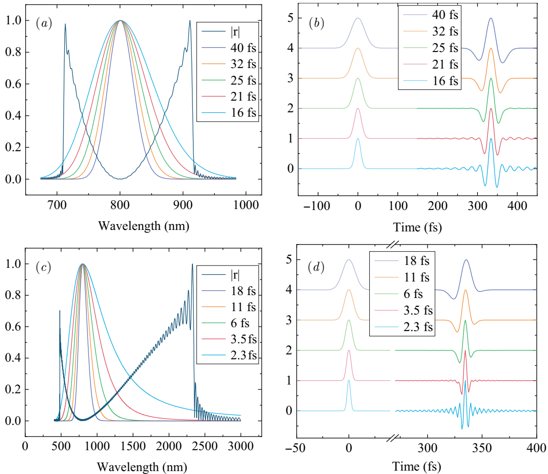
Рис. 7. Спектральные отклики дифференциаторов второго порядка с центральной частотой 12500\text{ см}^{-1} и шириной рабочего диапазона 3125\text{ см}^{-1} (a) и 16400\text{ см}^{-1} (c) и соответствующие им временные профили падающих (b) и отраженных (d) импульсов
