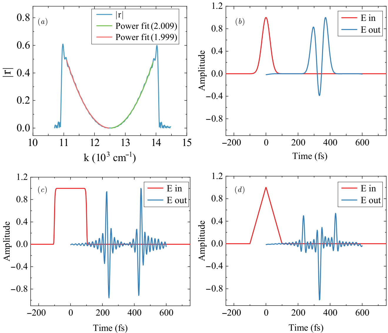
Рис. 3. Временные профили падающих и отраженных импульсов от ФК с линейно модулированной запрещенной зоной. Падающие импульсы: a — Эрмита – Гаусса 1 порядка, b — Эрмита – Гаусса 5 порядка, c — прямоугольный, d — треугольный
