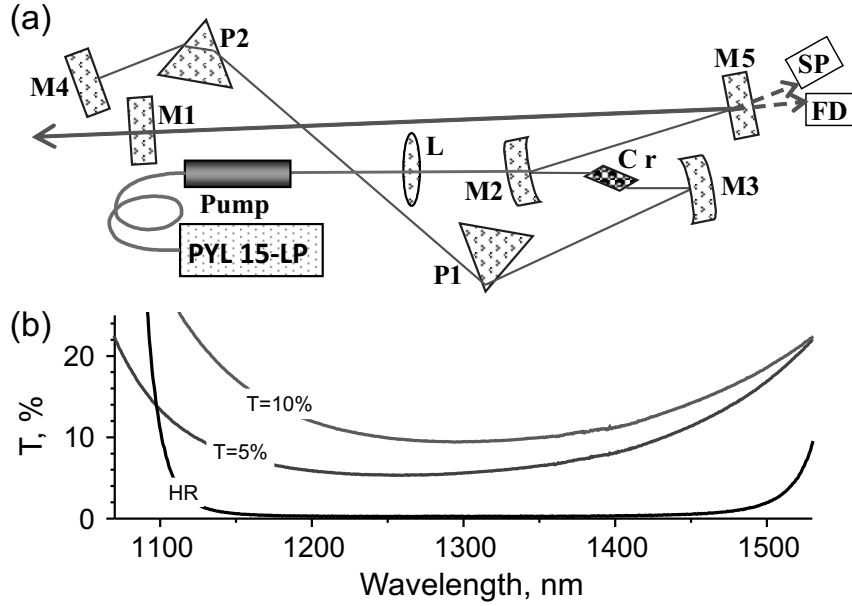
Рис. 1. a — Оптическая схема резонатора лазера: M1 — выходное зеркало, M2, M3 — сферические зеркала с радиусом кривизны 15 см; M4, M5 — плоские зеркала; P1, P2 — призмы из стекла SF14; Cr — кристалл \text{Mg}_2\text{SiO}_4:\text{Cr}^{4+} ; Pump — коллиматор иттербиевого волоконного лазера накачки PYL15-LP; L — линза излучения накачки с фокусным расстоянием 15 см; SP — спектрометр; FD — лавинный фотодиод ФД-2Г. b — Спектральные характеристики выходных зеркал 10%, 5% и 0.2%
