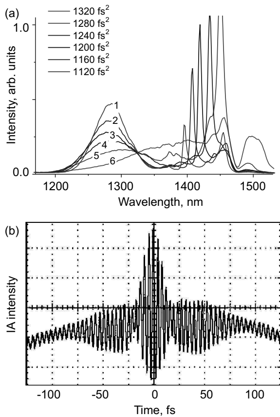
Рис. 5. a — Спектры излучения лазера хром-форстерита за ломающим зеркалом М5 (сплошные линии) с коэффициентом пропускания М1 0.2% при ДГЗ призм 1120 \text{fs}^2 (зеленая линии), 1160 \text{fs}^2 (голубая линия), 1200 \text{fs}^2 (синяя линия), 1240 \text{fs}^2 (бардовая линия), 1280 \text{fs}^2 (красная линии) и 1320 \text{fs}^2 (фиолетовая линии). b — Интерференционная автокорреляционная функция импульса при дисперсии призм 1280 \text{fs}^2
