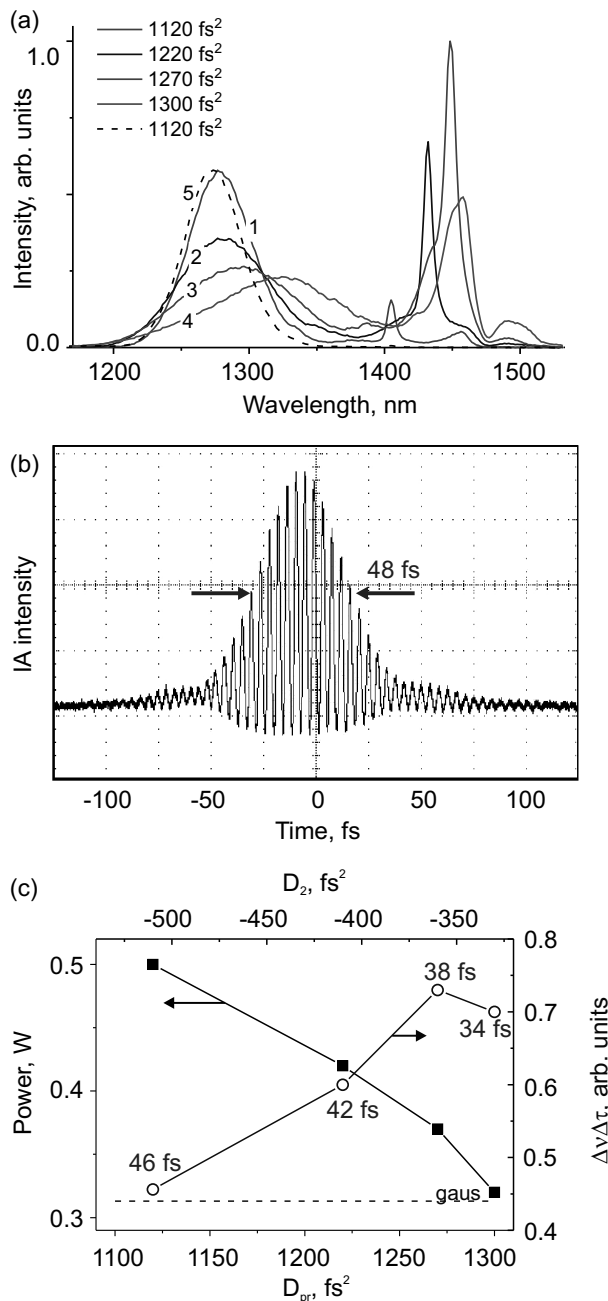
Рис. 4. a — Спектры излучения лазера хром-форстерита за глухим зеркалом М1 (штриховая линия) и ломающим зеркалом М5 (сплошные линии) с коэффициентом пропускания М1 5% при ДГЗ призм 1120 фс 2 (черная и зеленая линии), 1220 фс 2 (синяя линия), 1270 фс 2 (красная линия), 1300 фс 2 (фиолетовая линия). b — Интерференционная автокорреляционная функция интенсивности импульса (IA) при дисперсии призм 1300 фс 2 . c — Зависимости средней мощности и отношения \Delta\nu\Delta\tau импульсов от дисперсии резонатора
