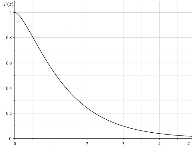
Рис. 1. График \mathcal{F}(z)
