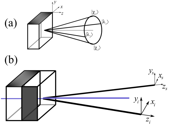
Рис. 4. a — Один из кристаллов двухкристальной схемы. Схематично показаны квантовые поляризационные состояния одиночных фотонов, соответствующие направлениям сбора в двухкристальной схеме. b — Оптическая схема источника — двухкристальная схема. Показано расположение скрещенных нелинейных кристаллов
