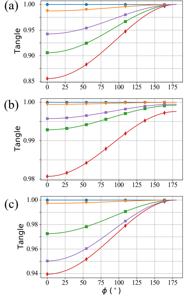
Рис. 5. Зависимости сцепленности (Tangle) от фазы \phi для кристалла ВВО (a), кристалла BiBO при \phi_p = 45^\circ (b), кристалла BiBO при \phi_p = 90^\circ (c). Синие кружки, оранжевые треугольники, зеленые квадраты, красные ромбы и пурпурные крестики соответствуют углам рассеяния 0^\circ , 3^\circ , 10^\circ , 17^\circ и 30^\circ снаружи кристалла. Соответствующие углы \theta_p приведены в таблице
