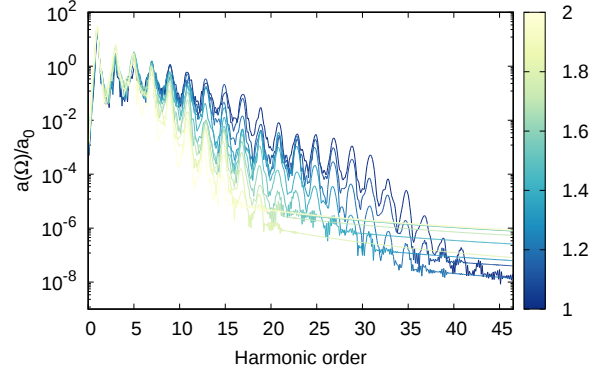
Рис. 2. (В цвете онлайн) Зависимость спектров ГВГ от номера гармоники представлена для C_{180} с использованием нормированного преобразования Фурье дипольного ускорения, a(\Omega)/a_0 , построенного в логарифмическом масштабе. Интенсивность волны равна 10 ТВт/см². Цветная полоса показывает частоту волны накачки в единицах \text{эВ}/\hbar
