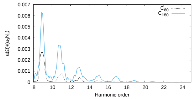
Рис. 6. Сравнение сигналов ГВГ, нормированных на число частиц, для C_{180} и C_{60} . Частота волны накачки равна \omega = 1.5 эВ/ \hbar (длина волны 827 нм), интенсивность волны 10 \text{ ТВТ/см}^2
