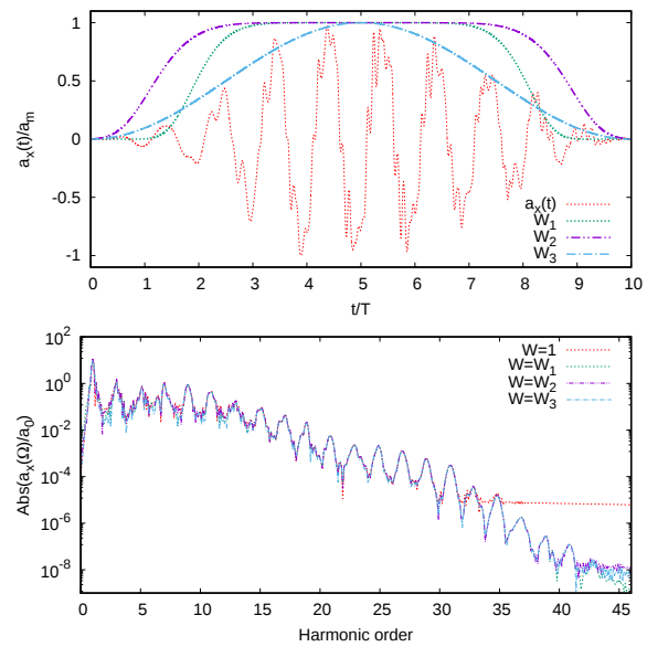
Рис. 7. (В цвете онлайн) На верхней панели изображена зависимость x -компоненты дипольного ускорения от времени вместе с оконными функциями. Интенсивность волны 10 \text{ ТВТ/см}^2 , частота 1 эВ (длина волны 1240 нм). На нижней панели показан спектр ГВГ, рассчитанный с использованием оконных функций, соответствующих дипольному ускорению на верхней панели
