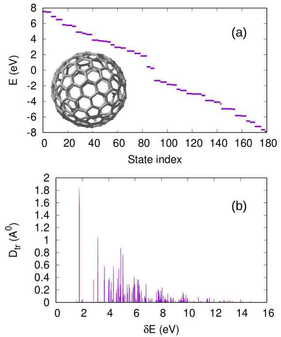
Рис. 1. a — Собственные энергии молекулы фуллерена C_{180} и b — модуль матричных элементов дипольного момента при межзонных переходах. На вставке приведена схематическая структура C_{180}
